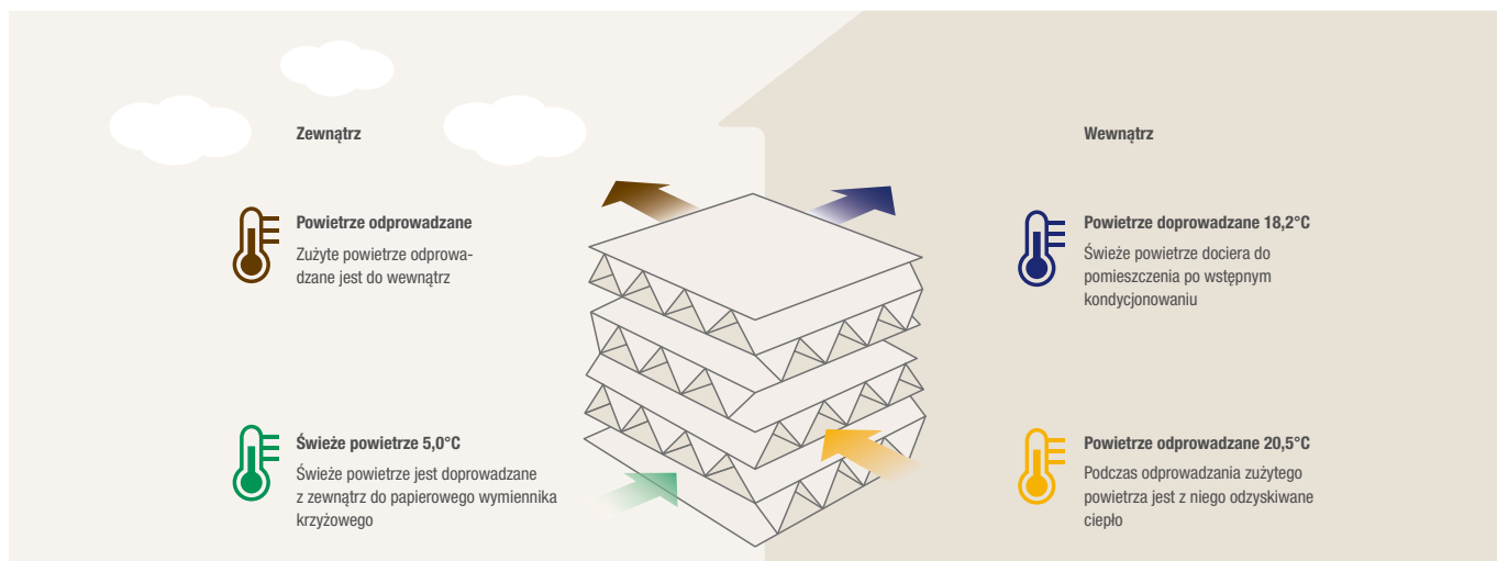
Struktura papierowego krzyżowego wymiennika ciepła Lossnay
