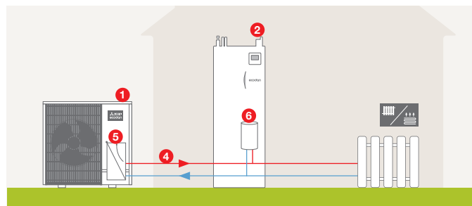
1 Unité extérieure 2 Unité intérieure 3 Tuyau de refroidissement 4 Conduite d'eau chaude (isolée) 5 Échangeur de chaleur à plaques 6 Chauffage de l'eau sanitaire
