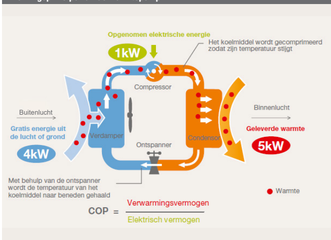
Werkingsprincipe van de warmtepomp
