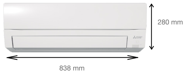
Afmetingen (B x H x D) voor de vermogens van MSZ-FT25-50VGK
