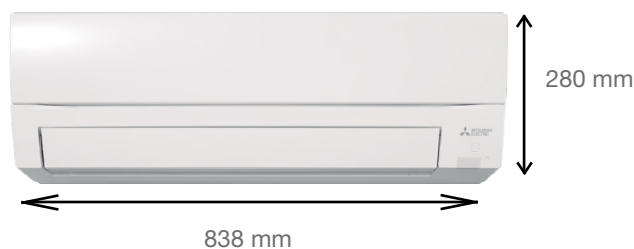
Dimensions (L x H x P) pour les capacités de MSZ-FT25-50VGK
