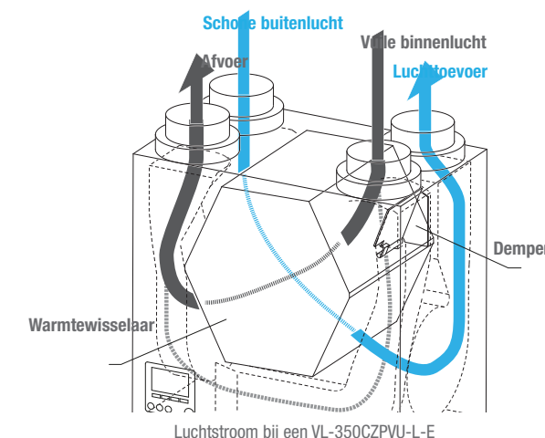
Luchtstroom bij een VL-350CZPVU-L-E
